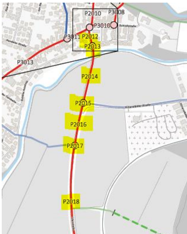
Abbildung 7 Maßnahmen des Pakets Verbindung Büdesheim - Kilianstädten
