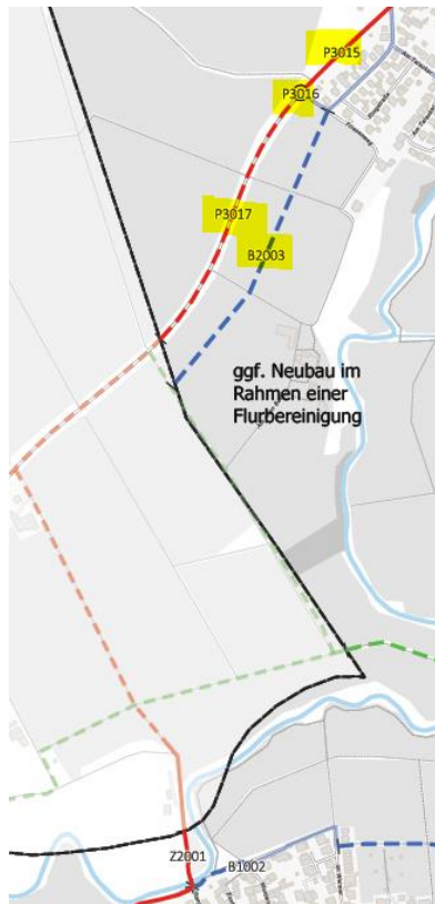
Abbildung 11 Maßnahmen B521 Richtung Süden
